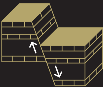
falla normal
