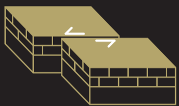
falla transformant
