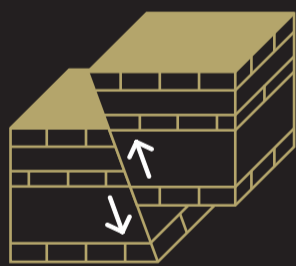
falla inversa
